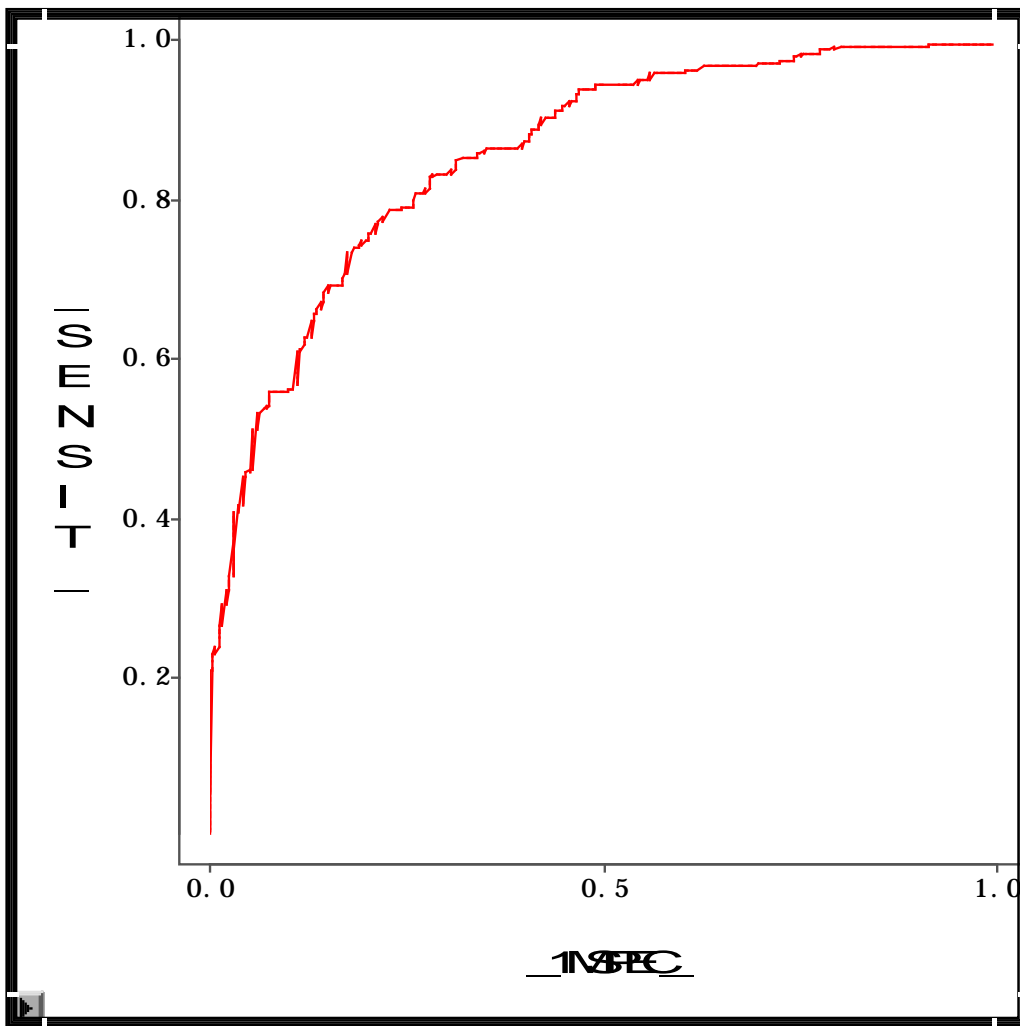
Courbe ROC
