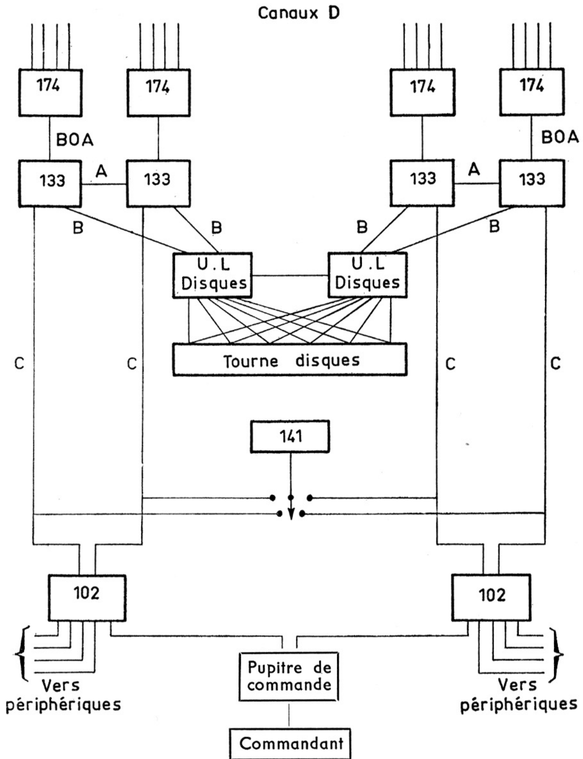
Figure 5 Schéma du centre de traitement des données
