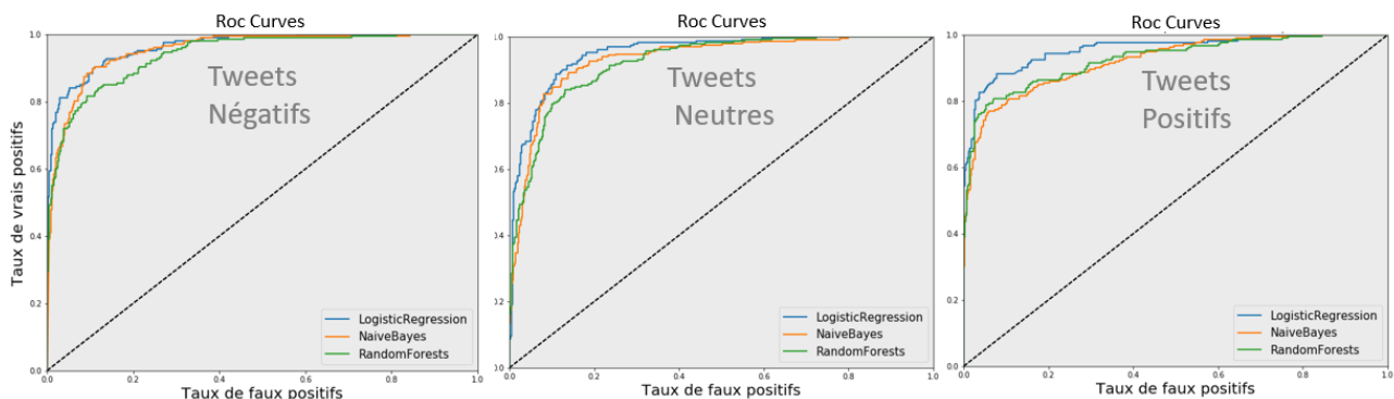
Figure 17: Comparaison des courbes ROC pour plusieurs modèles
