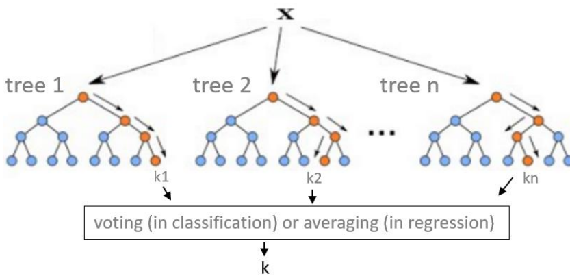
Figure 13: Algorithme des forêts aléatoires
