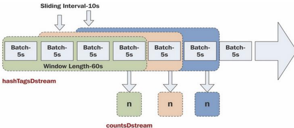
Figure 4: Opérations de fenêtrage avec Spark Streaming
