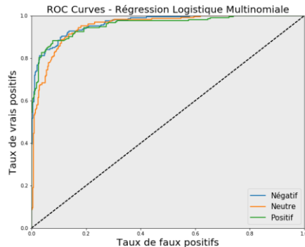
Figure 18: Superposition des courbes ROC de la Régression Logistique Multinomiale
