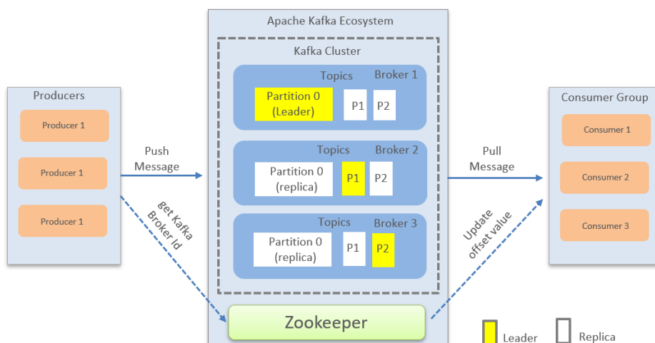
Figure 25: Passage à l'échelle de Kafka
