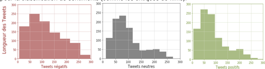
Figure 8 : Histogramme des longueurs des tweets selon le sentiment exprimé
