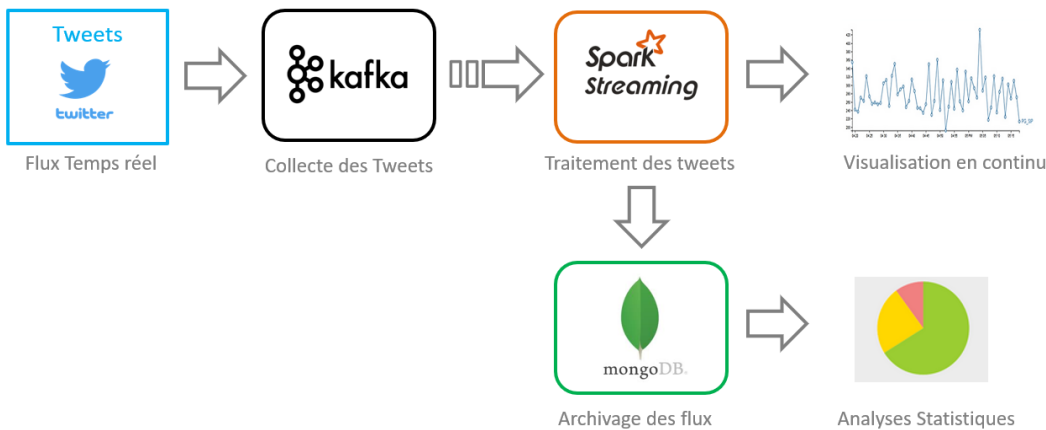
Figure 21: Architecture générale du projet
