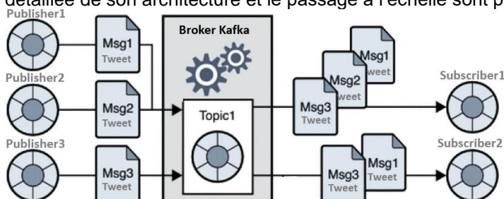
Figure 2: Système de messagerie Kafka
