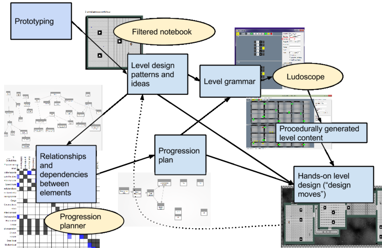
Figure 11 : flux du travail de conception de The Casimir Effect
