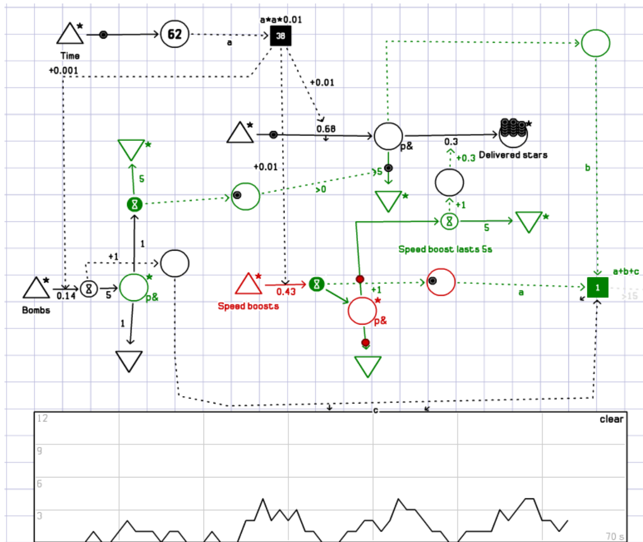
Figure 10 : la dynamique (en bas) simulé de la mécanique (en haut) de Ultraworm dans Machinations
